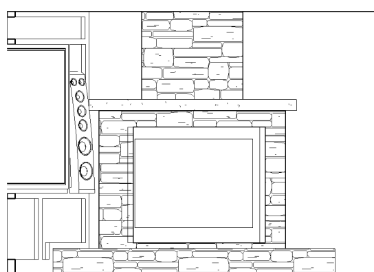
10 Elevation 2 - a A1 1/4" = 1'-0"
