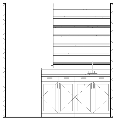
3 2 - c A1 1/4" = 1'-0"
