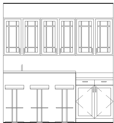
6 Elevation 1 - d A1 1/4" = 1'-0"
